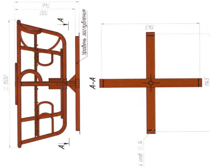
Рис. 4 – Общий вид.
